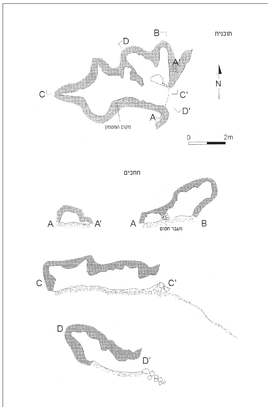
איור 9: תכנית וחתיכים של מערת צבר שבה נמצאו מטבעות הכסף
