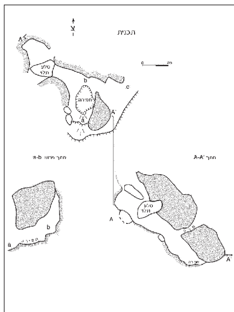
איור 16: כוך הלהבים (מערה 183), תוכנית וחתכים
