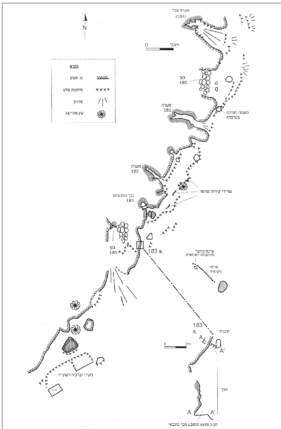
איור 4: התכנית של מכלול מערות צבר
