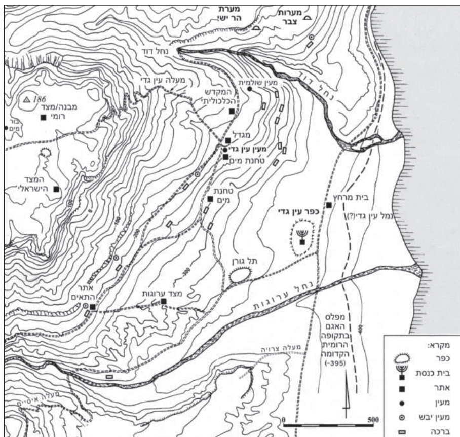
איור 2: נווה המדבר של עין-גדי בימי הבית השני, ומקום מערות צבר ומערת הר-ישי (על סמך Hirschfeld, 2007)
